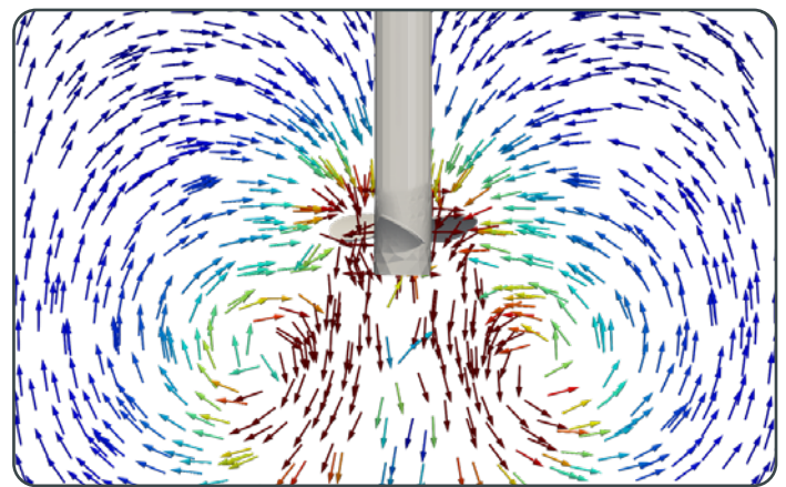
LÍNEAS DE FLUJO | REPRESENTACIÓN HÉLICE MARINA
