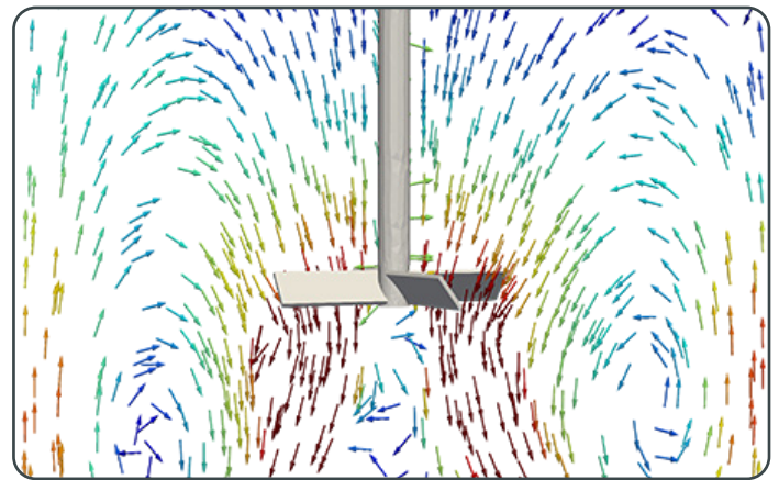
LÍNEAS DE FLUJO | REPRESENTACIÓN TURBINA AXIAL
